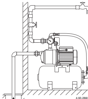
Fig. 2 Funzionamento in aspirazione Suction lift operation Saugbetrieb
